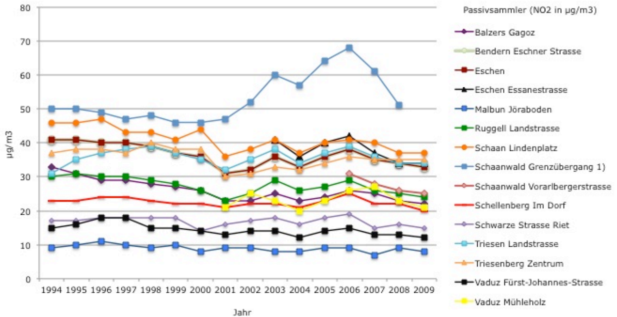
Abbildung 45: Passivsammler (NO 2 in µg/m 3 )
