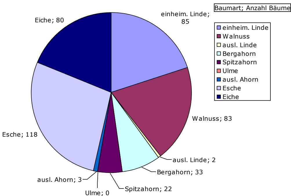
Abbildung 38: Vergleich der Baumartenauswahl 1999 und 2009
