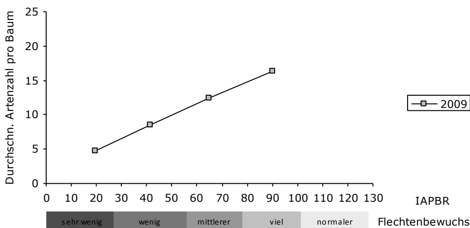
Abbildung 5: durchschnittliche Artenzahl pro Baum innerhalb einer Baumklasse
