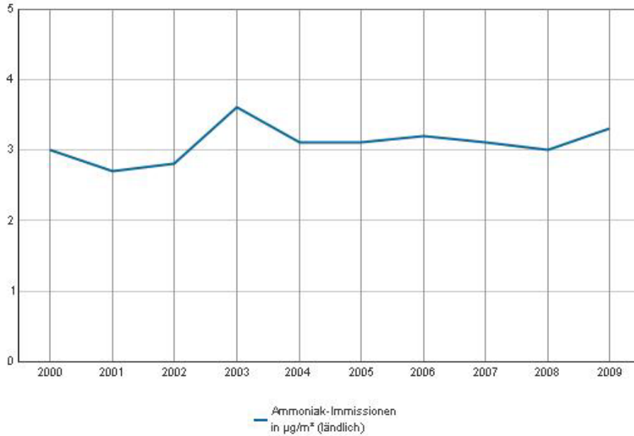
Abbildung 48: Verlauf der Ammoniakimmissionen von 2000 – 2009
