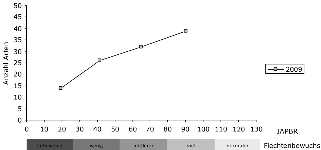
Abbildung 6: Artenvielfalt innerhalb einer Baumklasse
