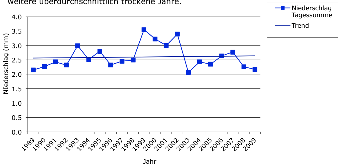
Abbildung 40: Verlauf des Niederschlages in Tagessummen wiedergegeben
