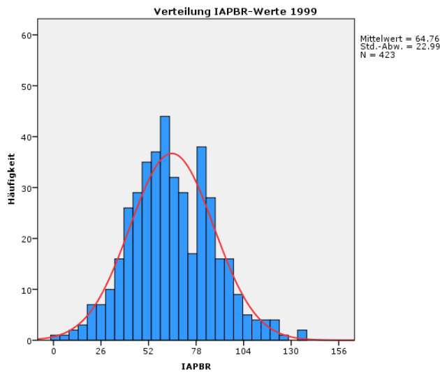
Abbildung 12: Verteilung der IAPBR-Werte 1999
