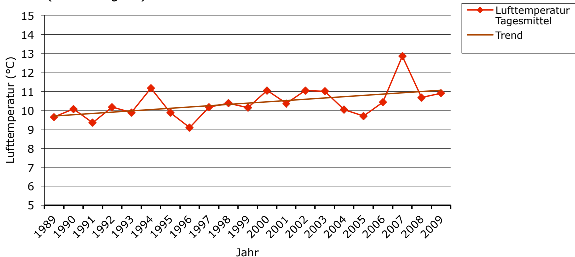
Abbildung 39: Verlauf der Tagesmittel der Lufttemperatur seit 1989 mit Trendlinie 13
