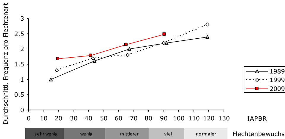
Abbildung 10: Durchschnittlichen Frequenz pro Flechtenart der Baumklassen im Vergleich
