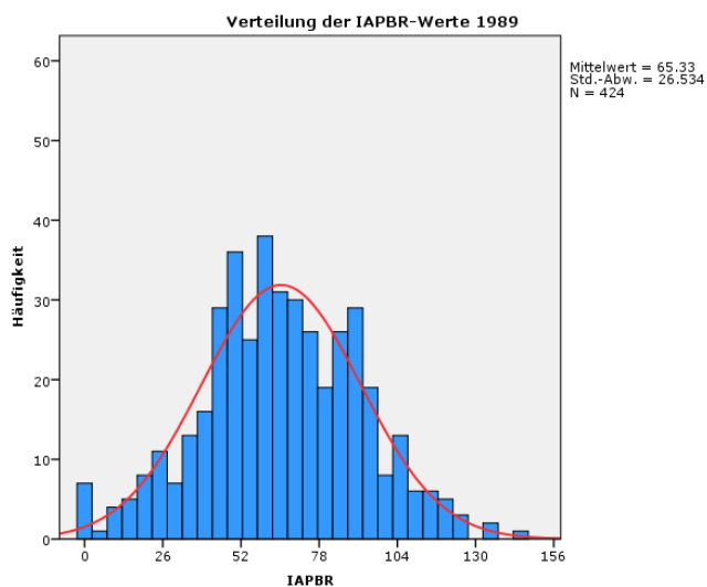
Abbildung 13: Verteilung der IAPBR-Werte 1989
