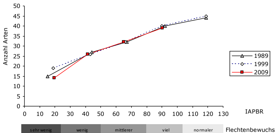
Abbildung 9: Artenvielfalt der Baumklassen im Vergleich
