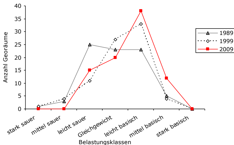
Abbildung 23: Verteilungen der Acidoindex in Richtung zunehmender basischer Belastung
