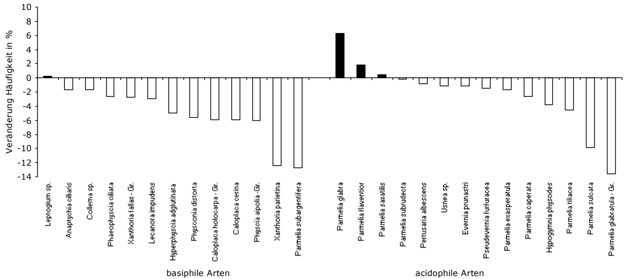
Abbildung 33: Veränderung der relativen Häufigkeit acidophiler und basiphiler Arten von 1999 bis 2009
