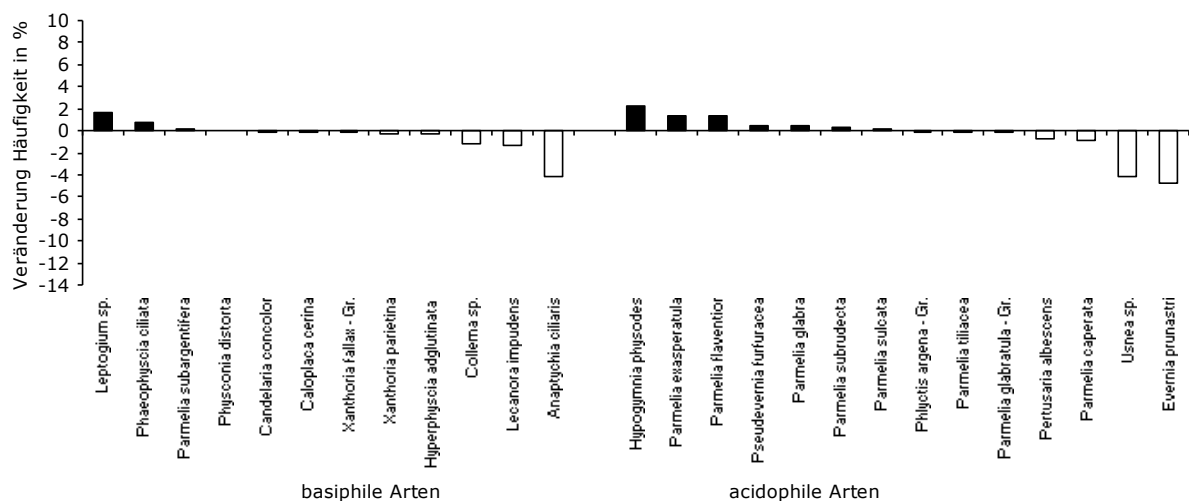
Abbildung 34: Veränderung der relativen Häufigkeit acidophiler und basiphiler Arten von 1989 bis 1999
