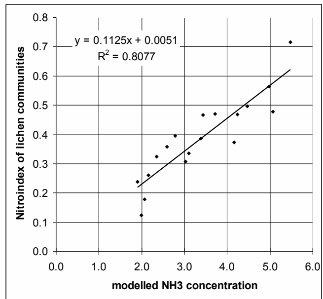
Abbildung 27: Zusammenhang zwischen Flechten-Nitroindex und modellierten NH 3 -konzentrationen (Jahresmittel Jahr 2000) (Abbildung aus Rihm et al. 2009)
