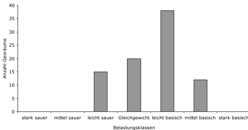
Abbildung 22: Vorkommen der Belastungsklassen im Jahr 2009
