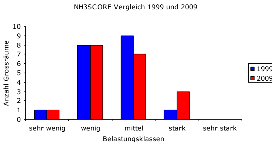
Abbildung 30: Vergleich der NH 3 SCOREs von 1999 und 2009
