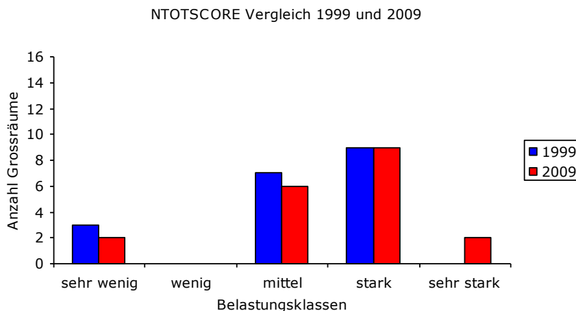
Abbildung 28: Verteilung der NTOTSCOREs 99 und 09
