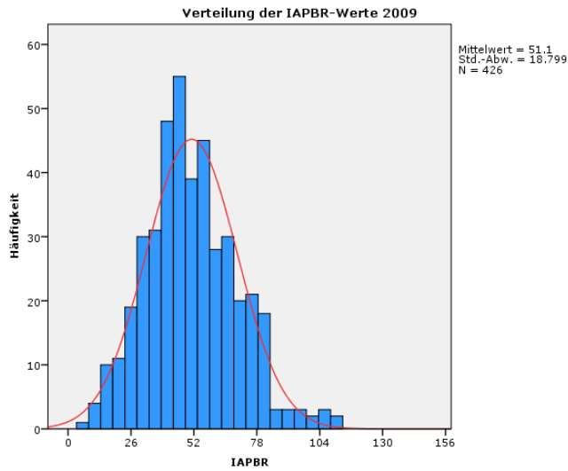
Abbildung 11: Verteilung der IAPBR-Werte 2009
