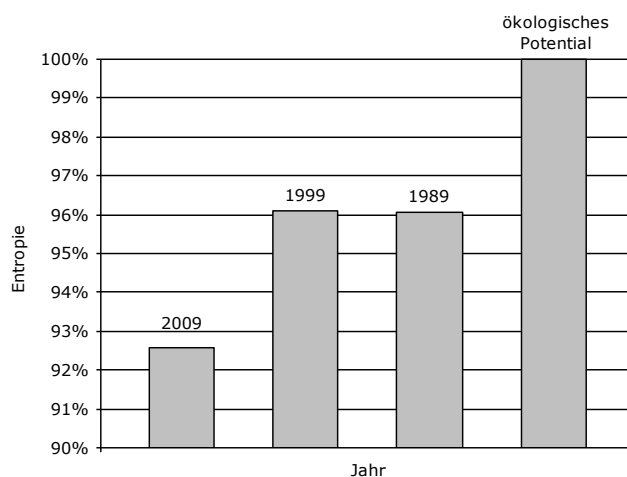
Abbildung 37 zeigt die Entropiewerte der Untersuchungen von 1989 bis 2009 in Prozent des maximalen Wertes (ökologisches Potential).
