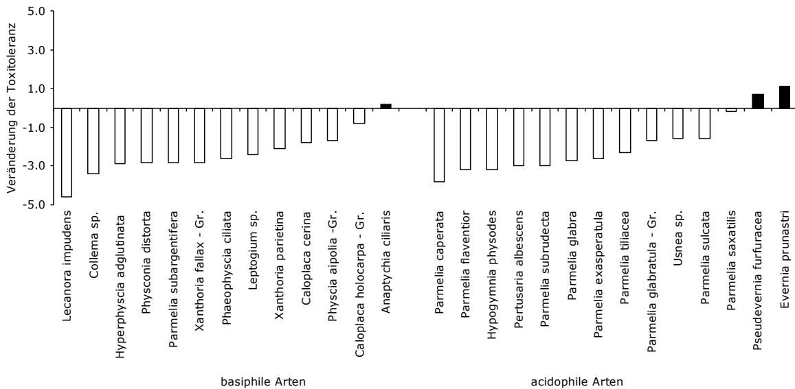
Abbildung 35: Veränderung des Toxitoleranzwertes von 1999 zu 2009 nach ökologischer Reaktionsweise geordnet
