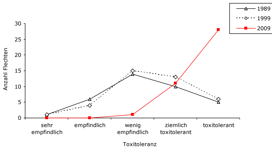
Abbildung 36: Vergleich der Toxitoleranz der Flechtenarten von 1989 bis 2009 bei mind. fünf (1%) Trägerbäumen (vgl. Tabelle 14)
