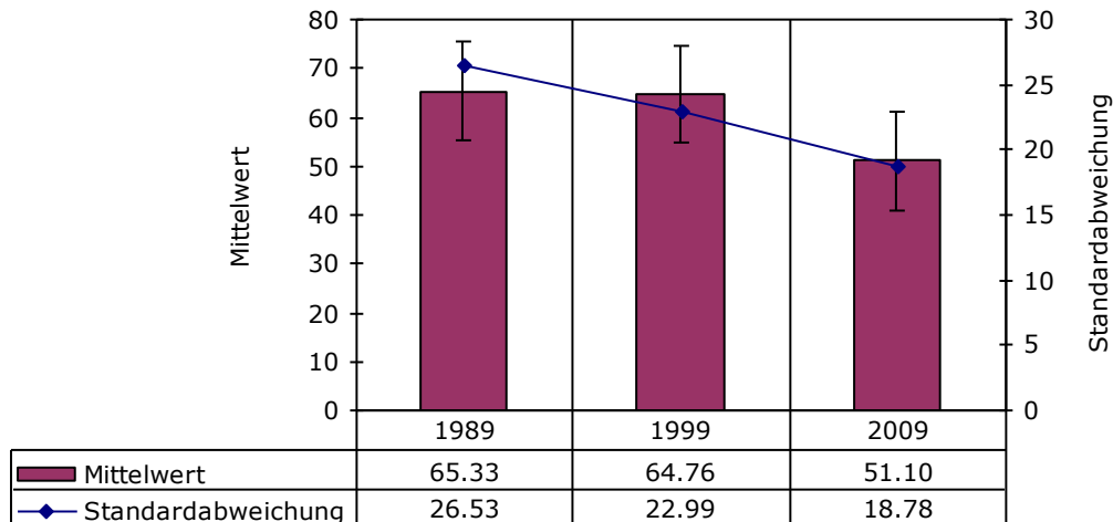
Abbildung 3: Vergleich der IAPBR-Mittelwerte und Standardabweichungen der Trägerbäume
