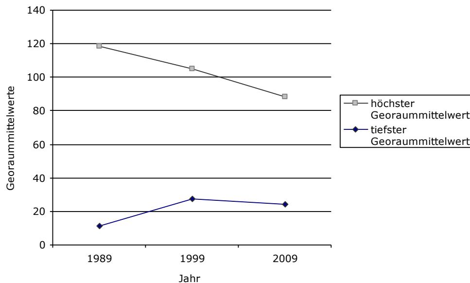
Abbildung 4 zeigt die höchsten und tiefsten IAPBR- Georaummittelwerte von 1989 bis 2009
