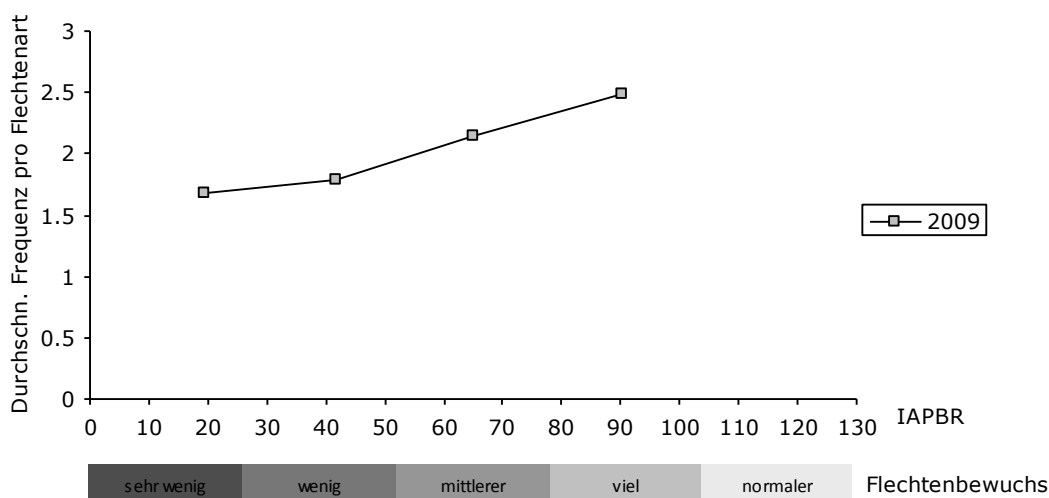
Abbildung 7: Durchschnittliche Frequenz pro Flechtenart 2009
