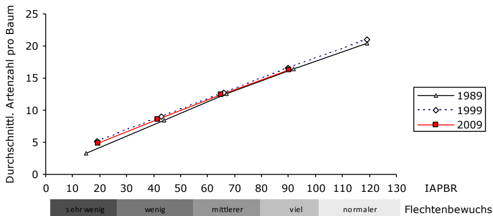
Abbildung 8: durchschnittliche Artenzahl pro Baum innerhalb einer Baumklassen im Vergleich
